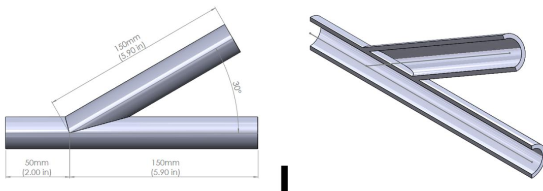
图B-39 防滚架焊样件二
