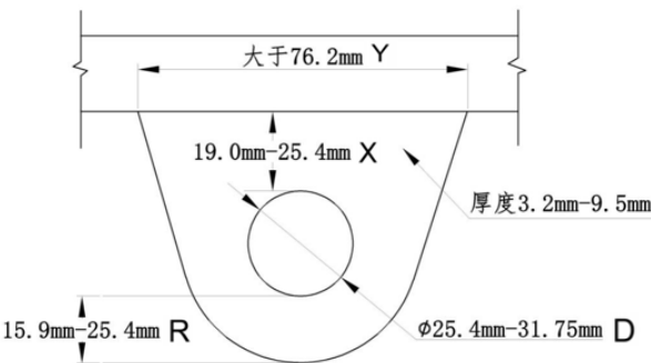
图 B-70 后拖拽点尺寸图
