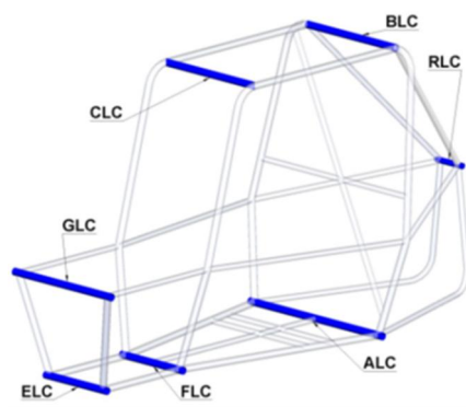
图 B-24 防滚架横向横梁 LC
