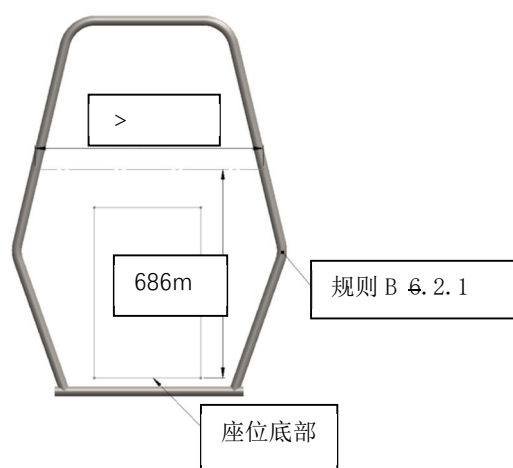
图B-25 防滚架 RRH
