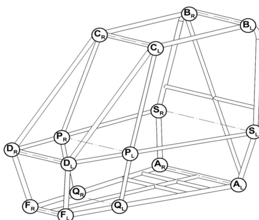
图B-23 防滚架示例、定义点、前支撑
