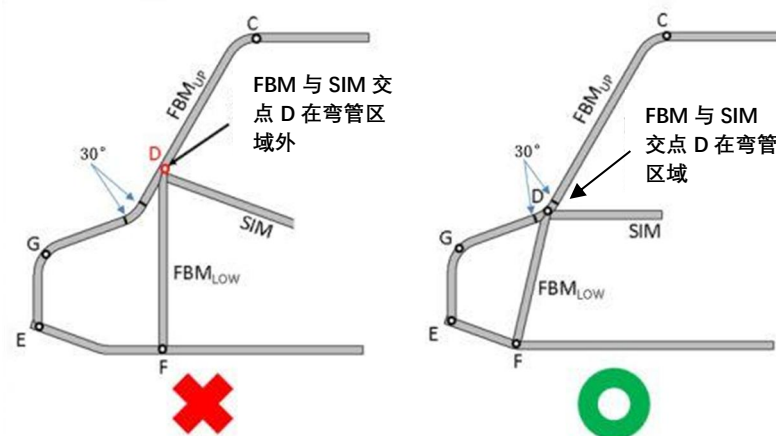
图B-19 防滚架弯管交点位置
