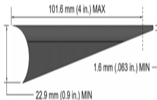
图 B-7 允许锥度
