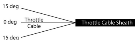
图B-10 油门拉索护套角度
