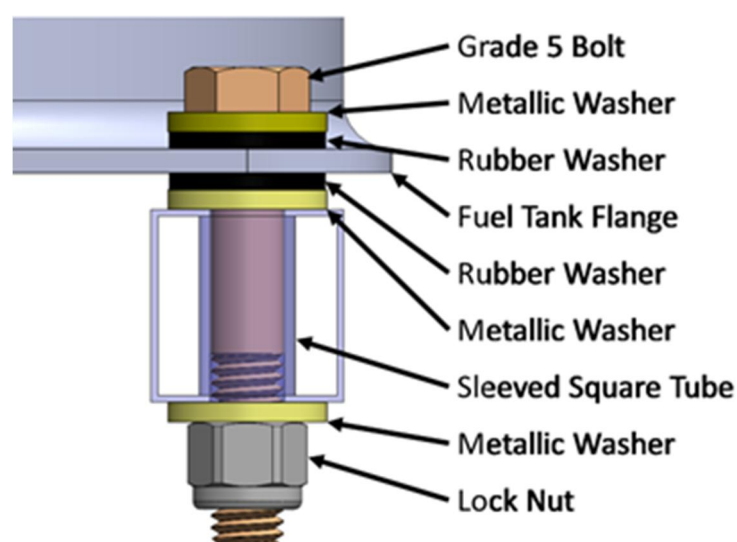
图B-4 油箱紧固件安装示意图
