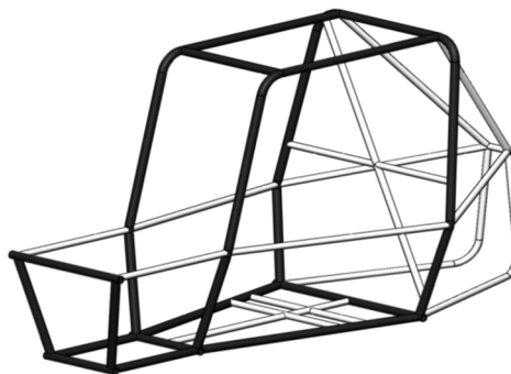
图B-21 防滚架主要构件(黑色填充)，后支撑车架
