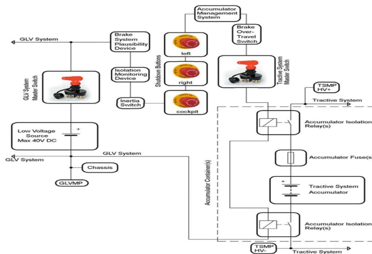
图B-12 安全回路原理图
