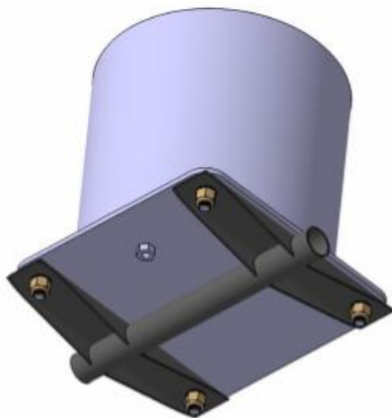
图B-6 安装在“C”支架上的油箱。(可接受安装方案)
