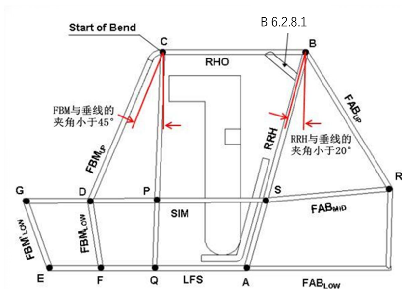
图B-34 防滚架FBM
