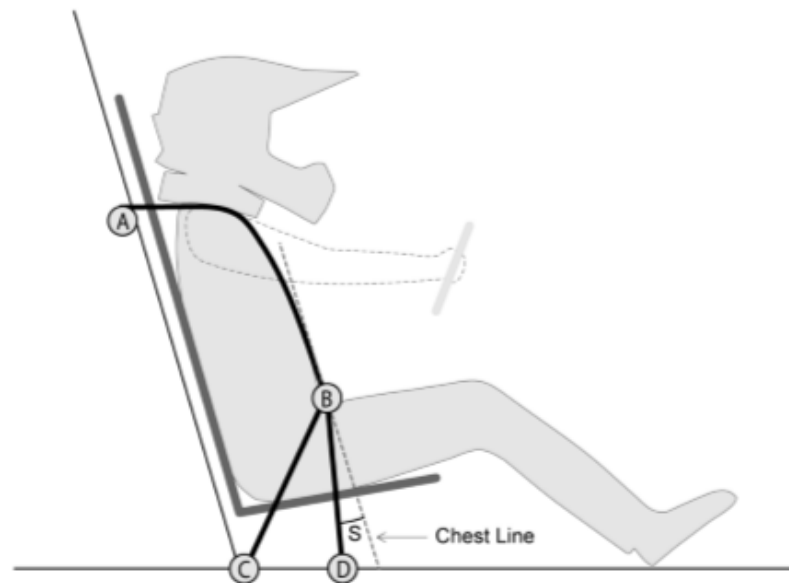
图B-52 车手安全带，反潜带角度
