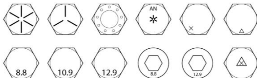
图B-71 紧固件，可接受的标记
