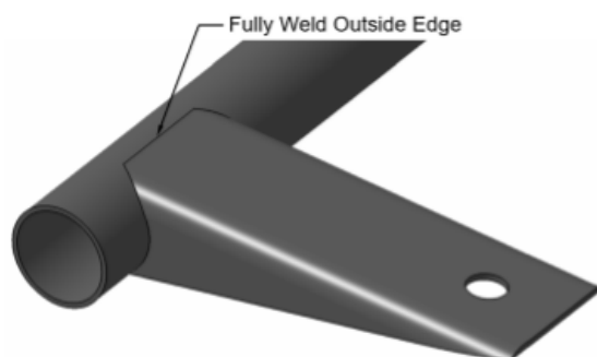
图B-8 最小焊接长度
