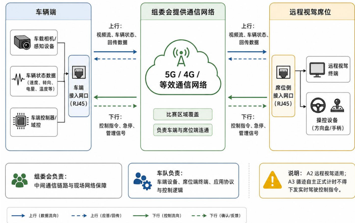
图3-1 远程视驾通信链路示意图
