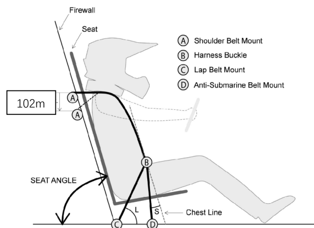
图B-43 安全带约束示意图
